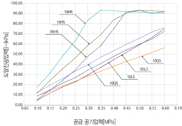
도달진공압력특성
