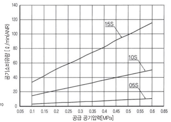
공기소비유량 특성
